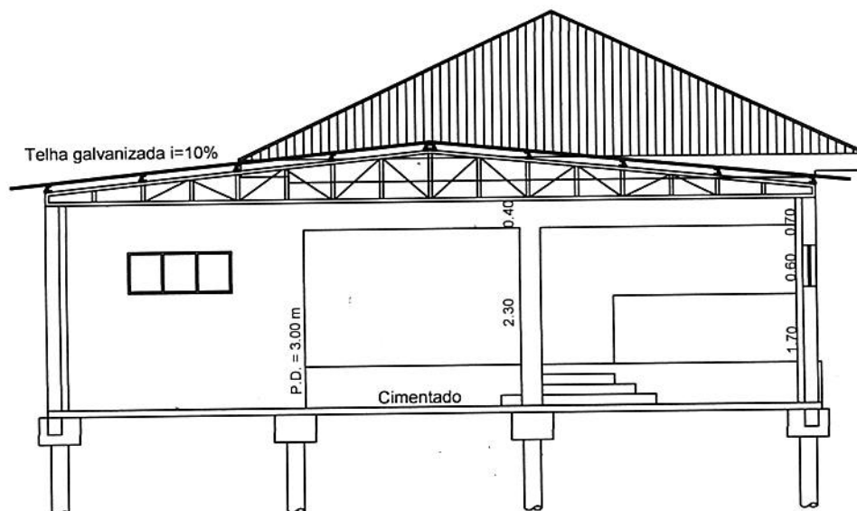
CORTE A-A Esc. 1 : 100
