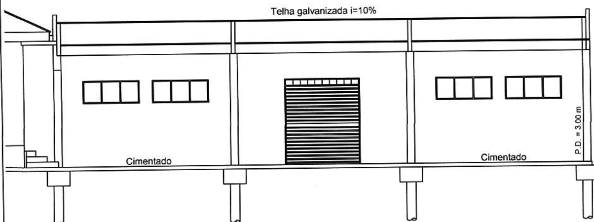
CORTE B-B Esc. 1 : 100
